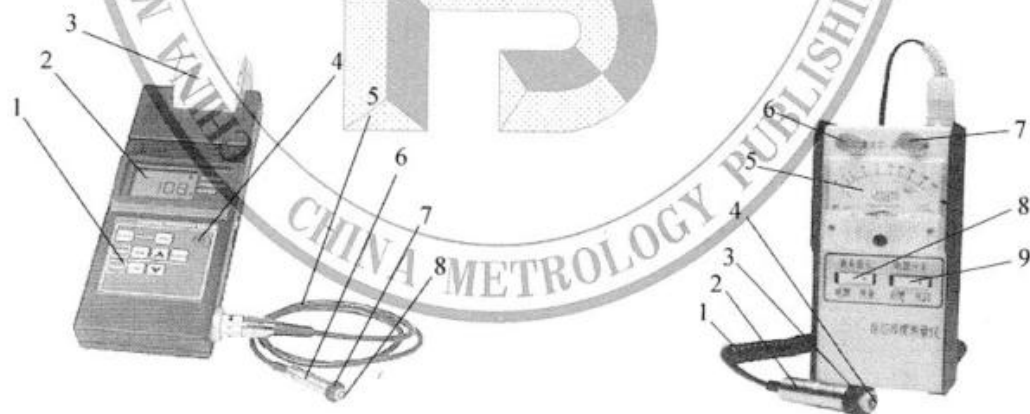
(a) 数字式覆层厚度测量仪外形图
