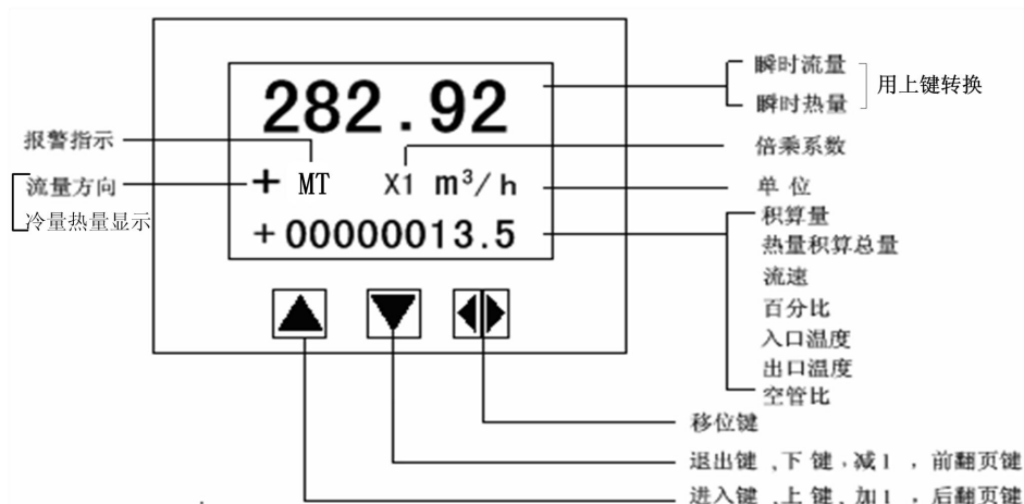
图 3.1 键盘定义与液晶显示
