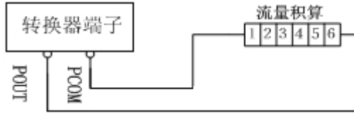
图 1.4 内供电源接电子计数器
