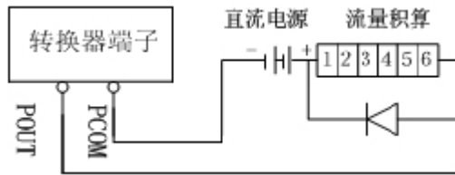
图 1.3 外供电源接电子计数器
