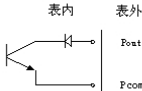
图 1.6 表内 OC 门连接方式
