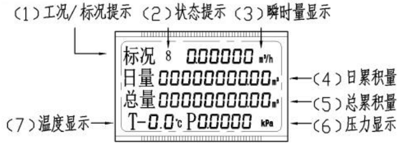
图 6-2 工作界面示意图
