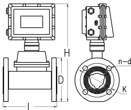
图 4-2 法兰连接示意图
