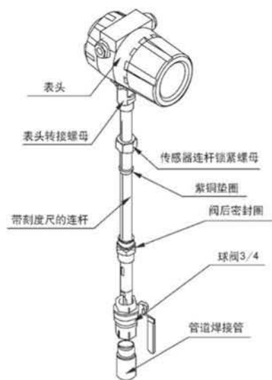
精简型热式气体质量流量计
