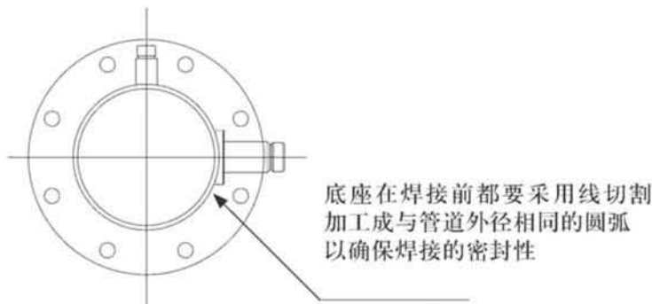
图4 理想底座焊接位置
