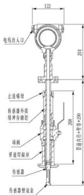
标准型热式气体质量流量计
